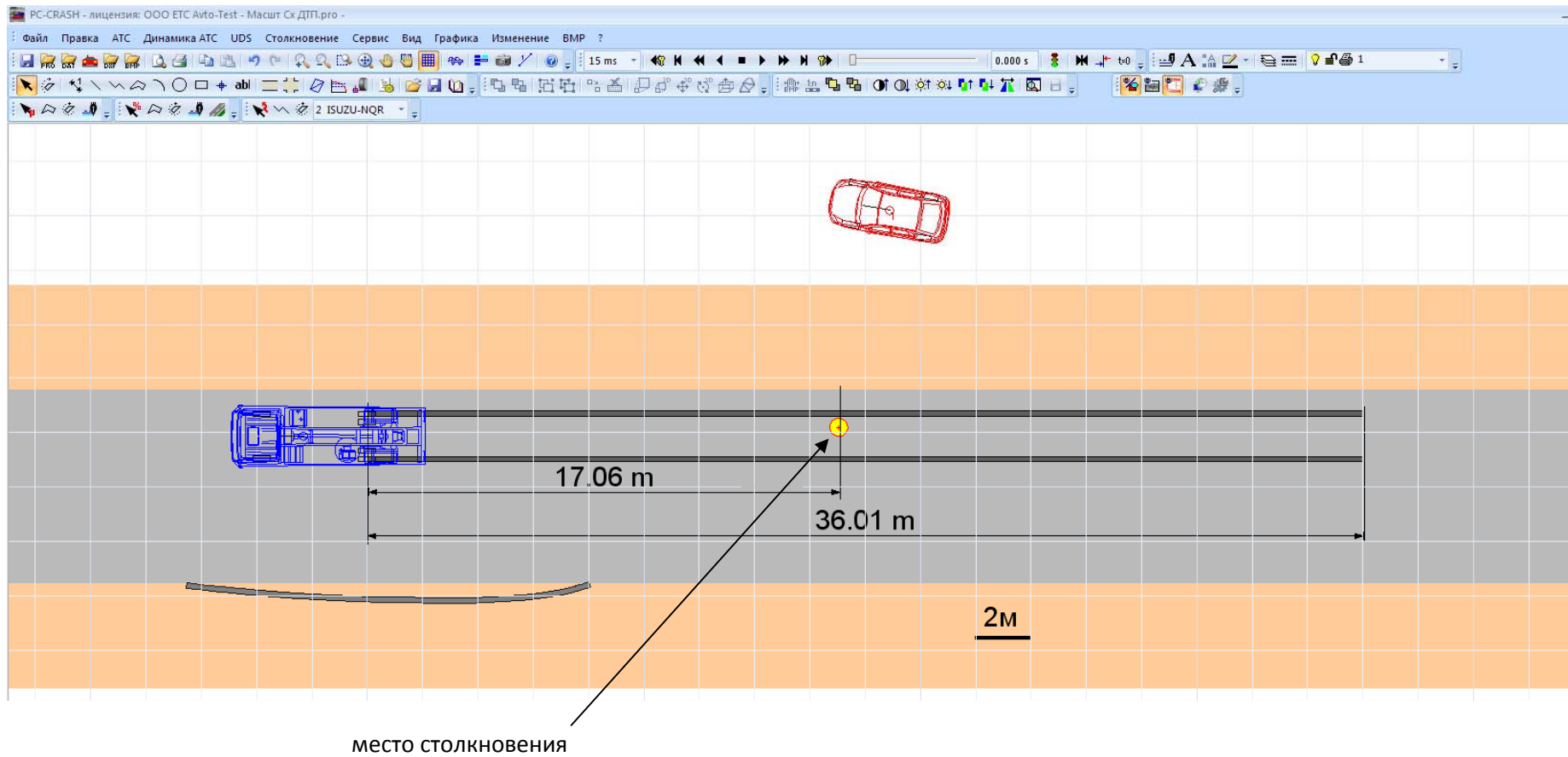
Рис.1. Масштабная схема ДТП.
