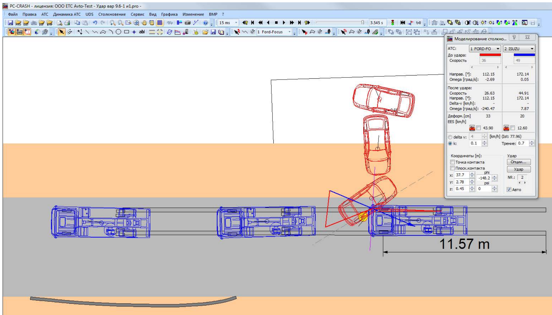
Рис. 2 Расчет столкновения. Масса груза Исудзу -6233 кг.
