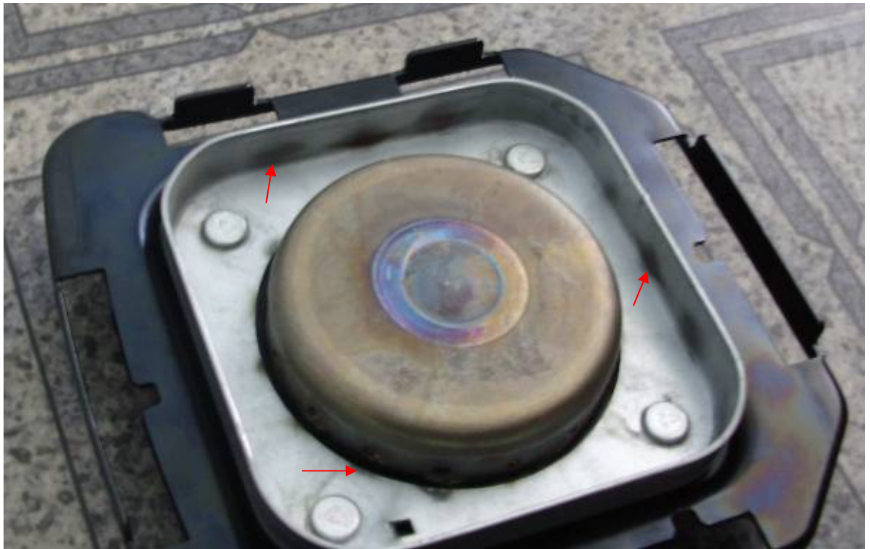
Фото 7. Внутренняя часть модуля подушки безопасности водителя с газогенератором на момент осмотра (стрелками указаны следы работы газогенератора в виде оскотченостей).
