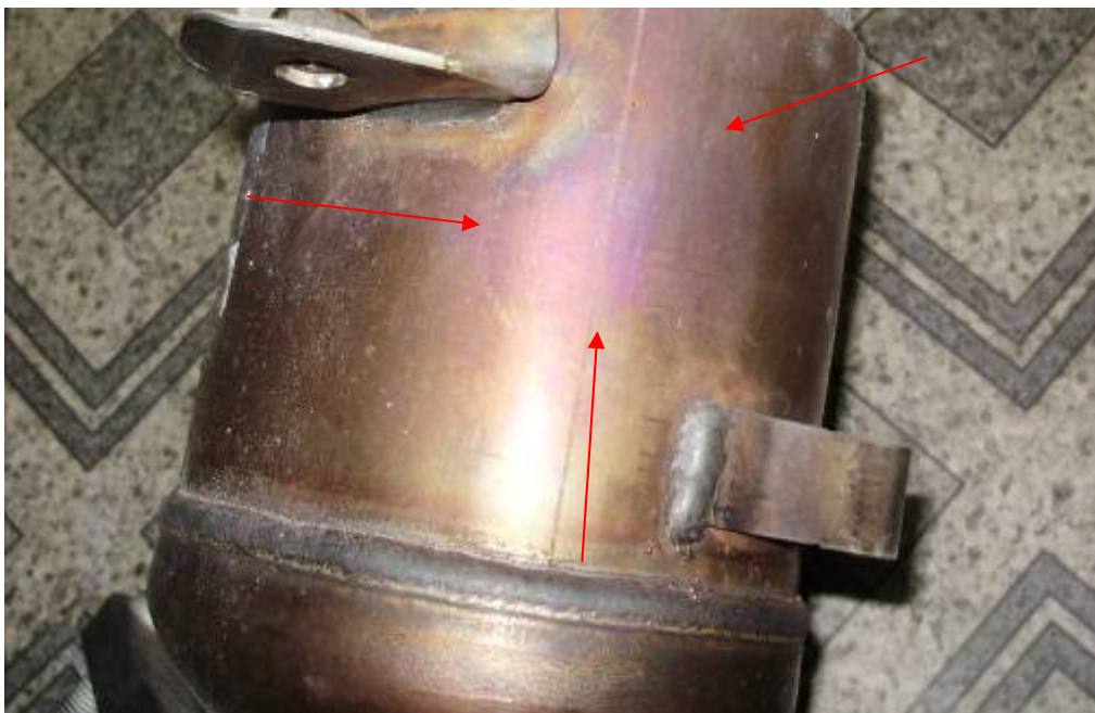
Фото 5. След побежалости на корпусе каталитического нейтрализатора.
